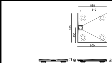
DW-RA-90-90: 900 x 900 mm
